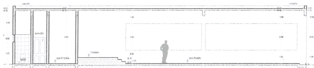
SECCIÓN A ESC. 1:50 EDIFICIO MULTIUSO
